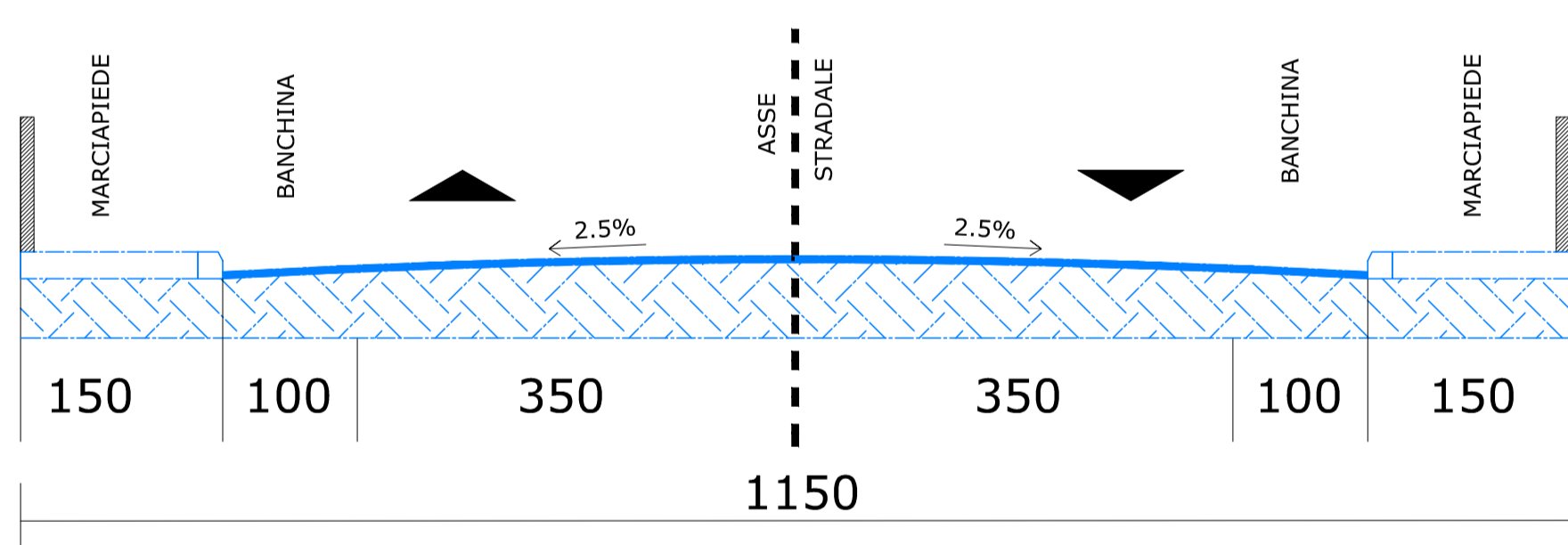
SEZIONE ASSE DI PENETRAZIONE DA ROTATORIA SU S.P.236 A ROTATORIA INTERNA
