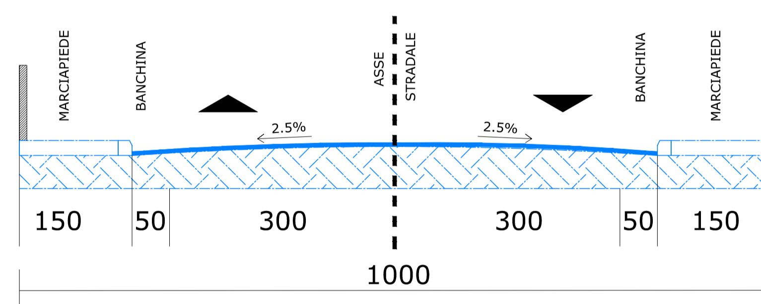
SEZIONE TIPO ASSE STRADALE INTERNO AL PIANO INSEDIAMENTI PRODUTTIVI ARTIGIANALE
